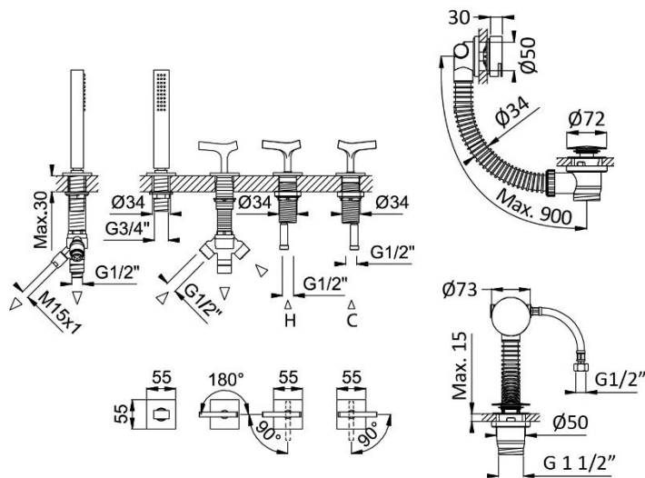
DESENHO DIMENSIONAL | DIMENSIONAL DRAWING
