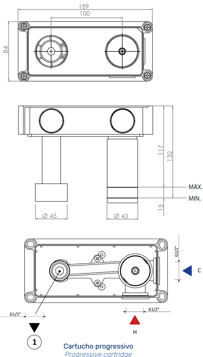
DESENHO DIMENSIONAL | DIMENSIONAL DRAWING
